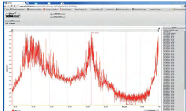
Surveillance en ligne du débit avec les données de l'appareil de mesure par ultrasons SebaFlow
